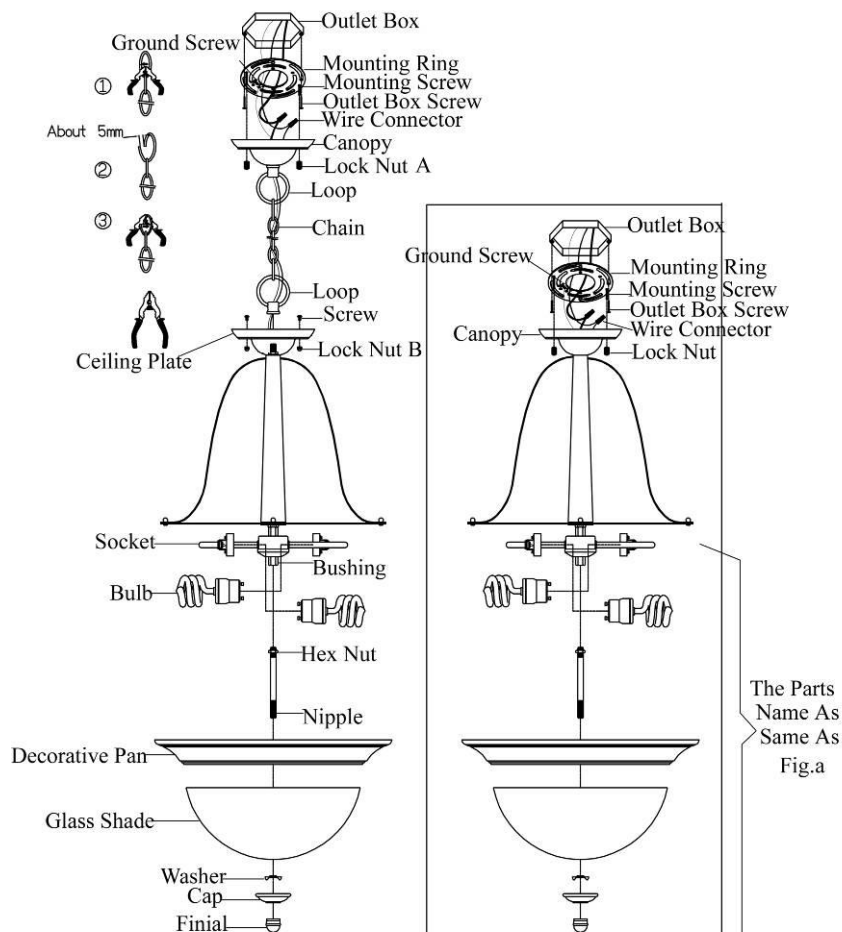
Fig.a: Install for Pendant
