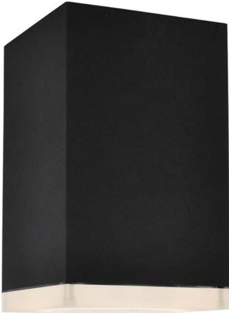
AV9888-BLK Black 4.7"W x 8"H x 4.7"EXT 14W / 120V 795 Lumens 3000K
