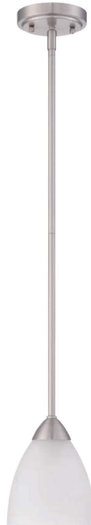
37791-SN - 1 Light Mini Pendant 5.75"W x 7"H; 3 x 12" & 1 x 6" Downrod; 10' Wire 60 Watt Medium Base; White Frosted Glass - 5.75"D
