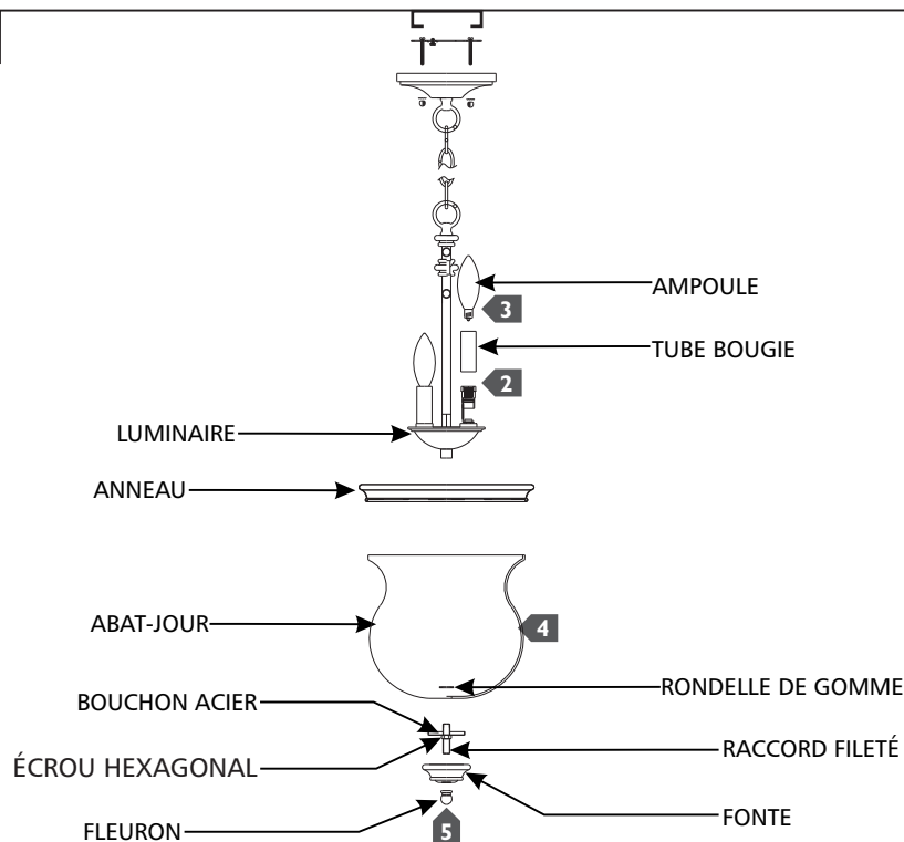
INSTALLATION DE MONTAGE SEMI-ENCASTRÉ
