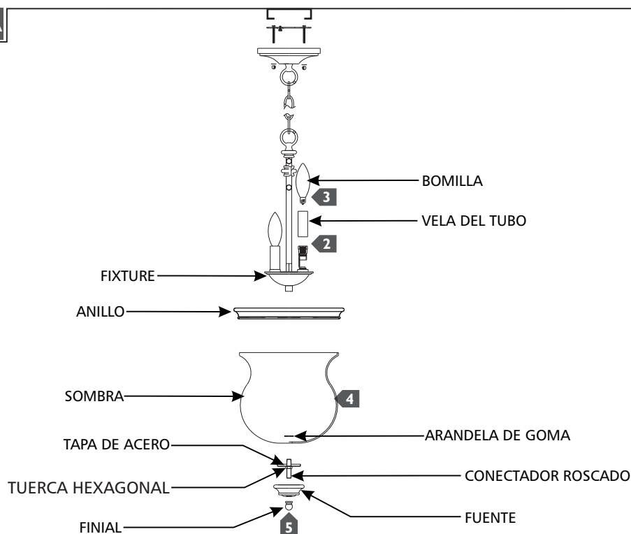
INSTALACIÓN DE SEMI-FLUSH MOUNT
