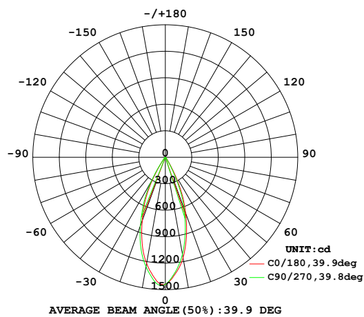
32° Beam Angle - 2700K (90 CRI)
