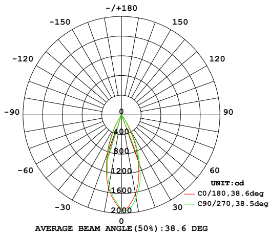
32° Beam Angle - 2700K (85 CRI)
