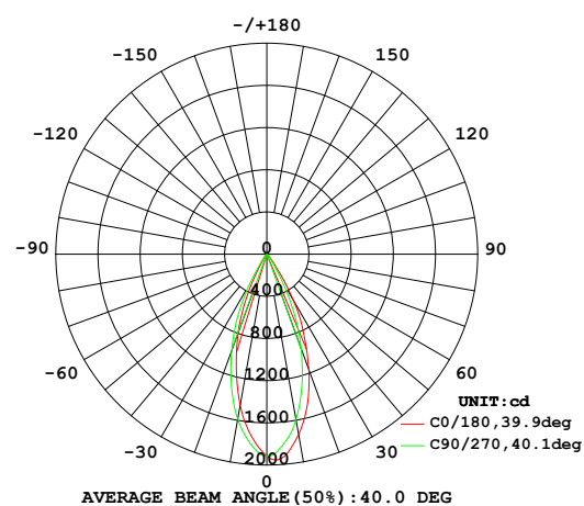
32° Beam Angle - 3000K (85 CRI)
